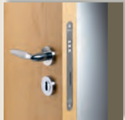
MAGNETSCHLOSS für stumpf einschlagende Elemente
